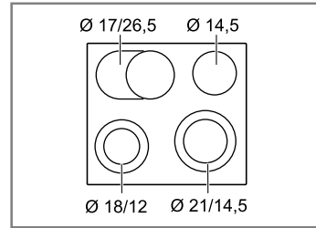
ET6FNP..
