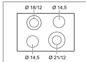
ET7..FGP1.
